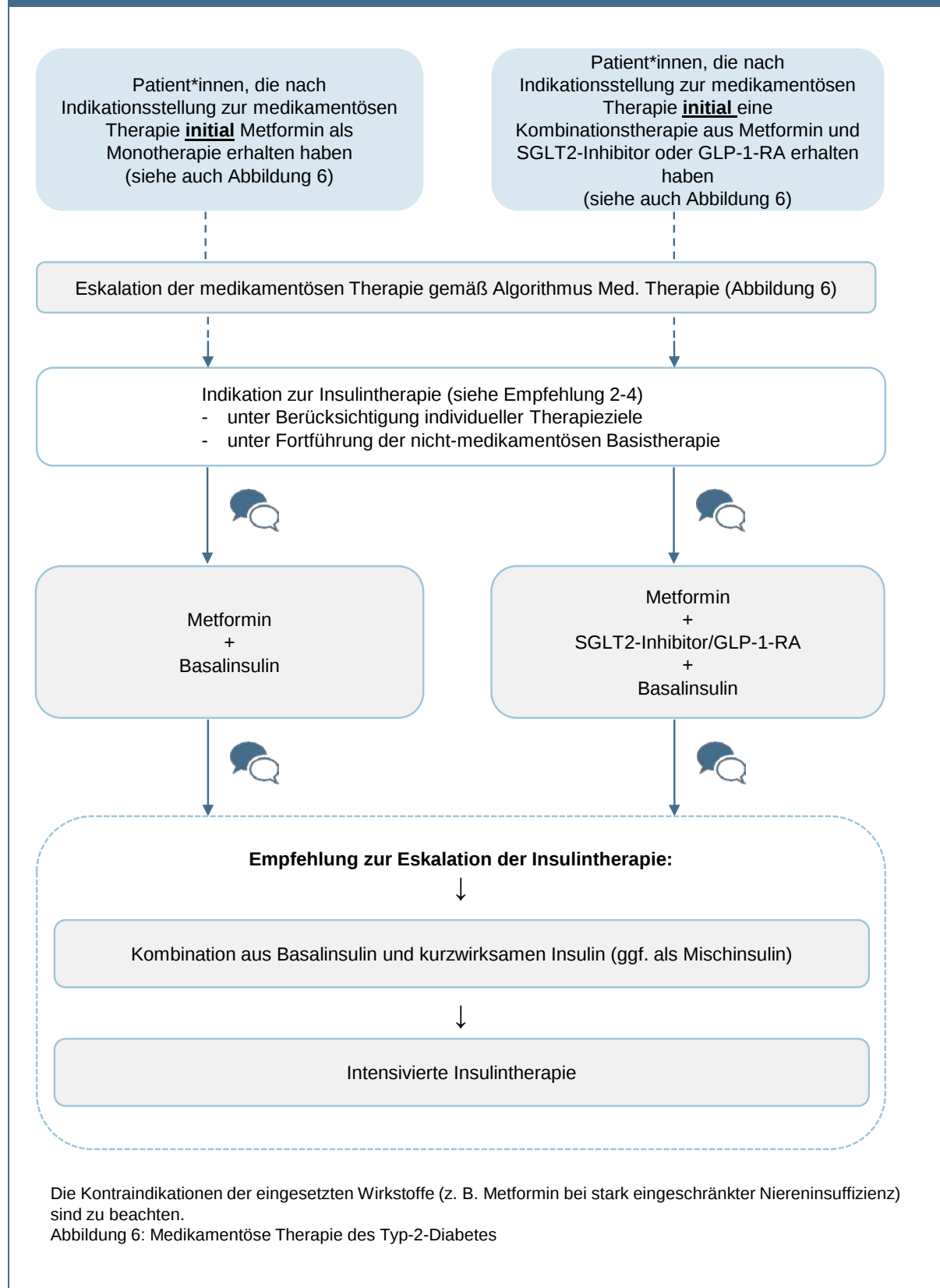
Abbildung 7: Algorithmus Insulintherapie
